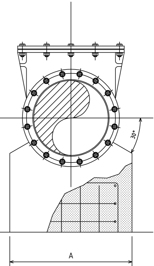
END ELEVATION
